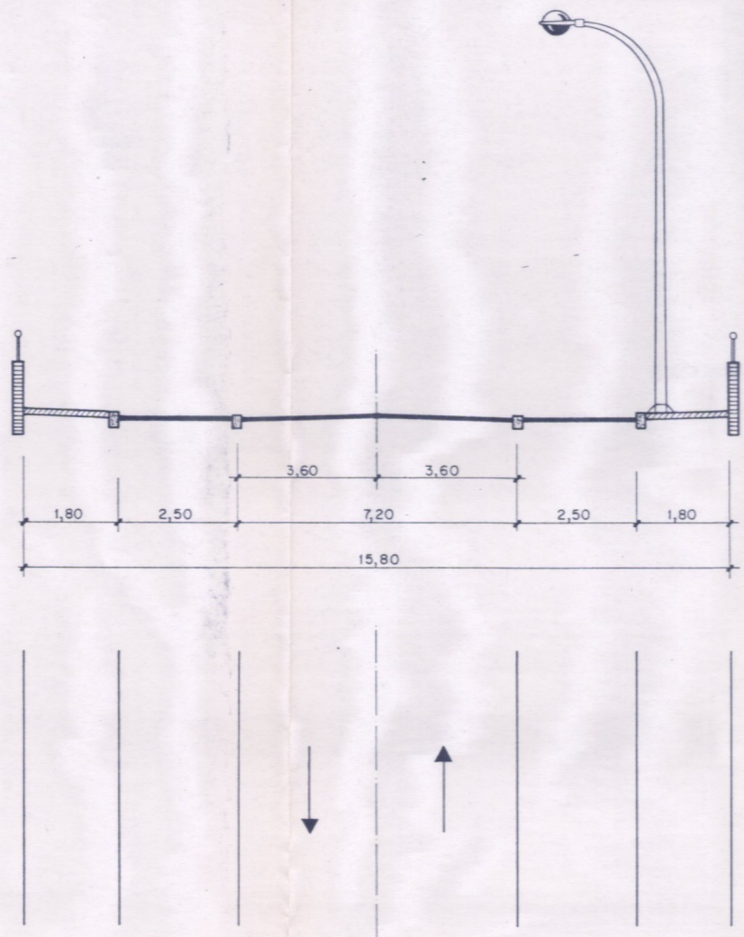
CALLE DE 15,80 (CALLES B,C y D)
