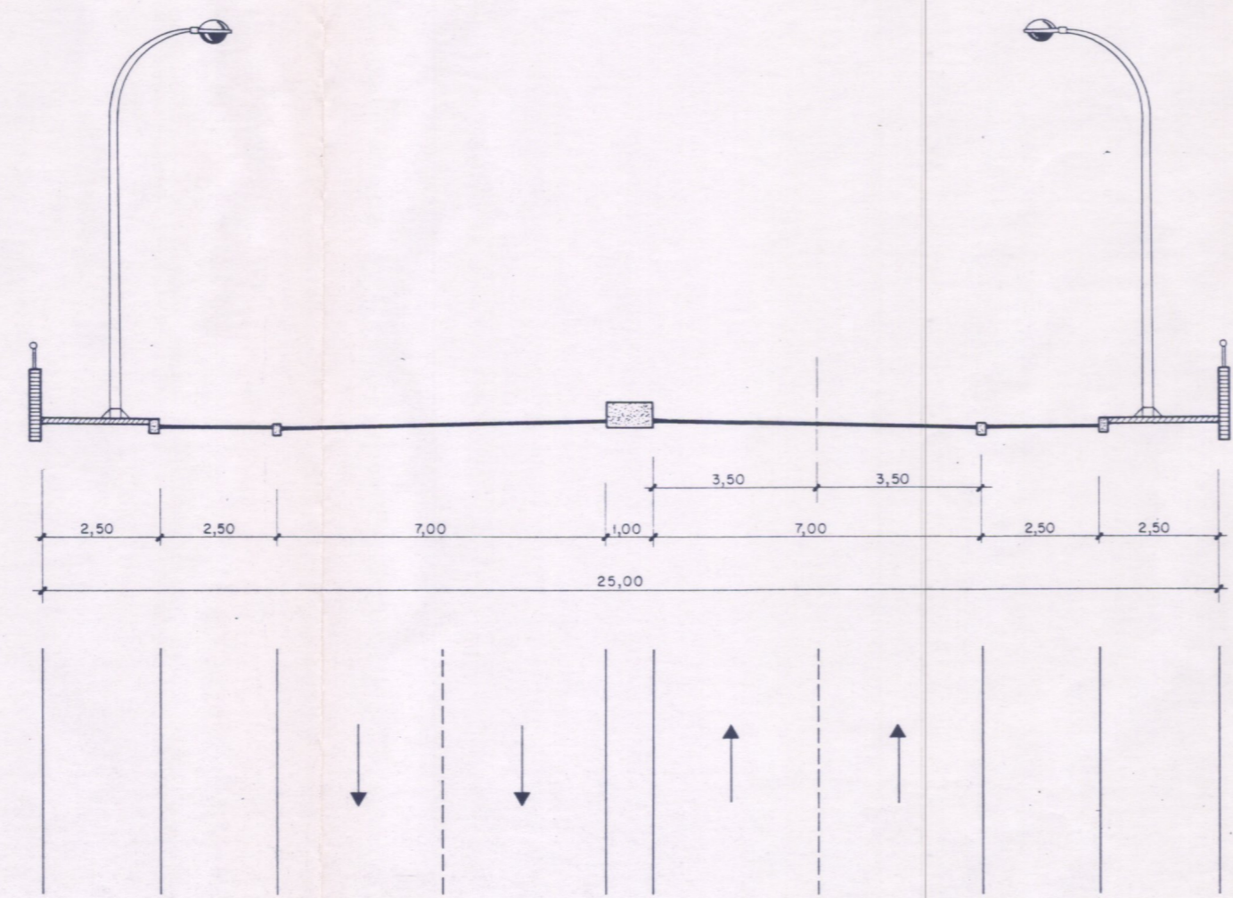
CALLE DE 25 m. (CALLE A)
